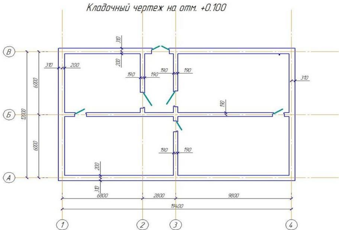
Рисунок 1. Кладочный чертеж
